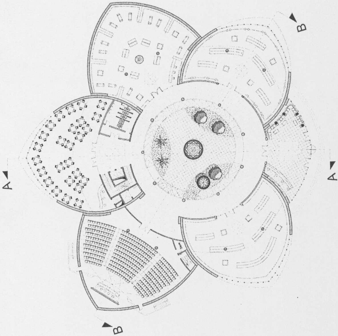
مسقط الطابق الأرضي
